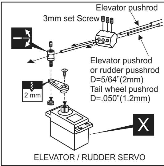
FUSELAGE BOTTOM-VIEW UNTERSICHT
