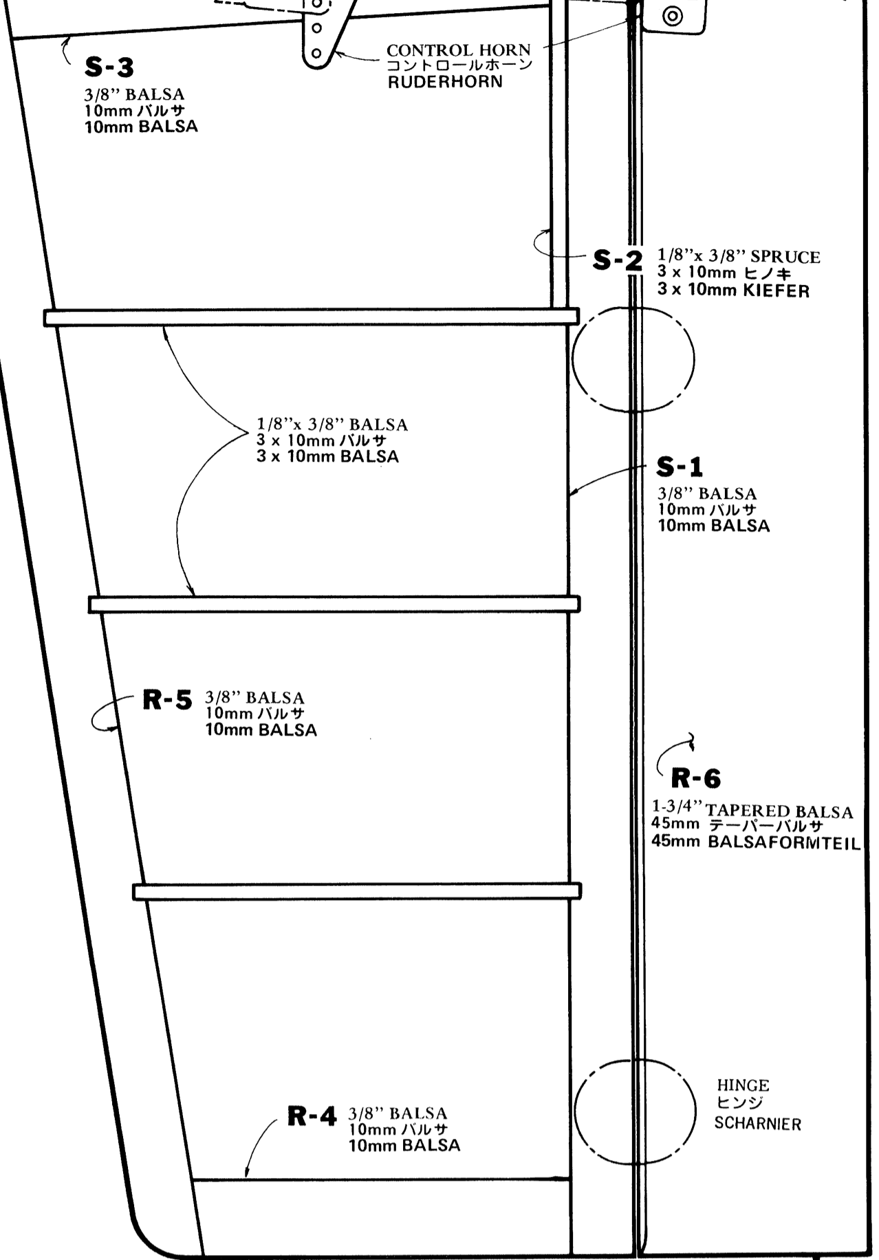
STABILIZER TOP VIEW 尾翼上面図 HÖHENRUDER VON OBEN
